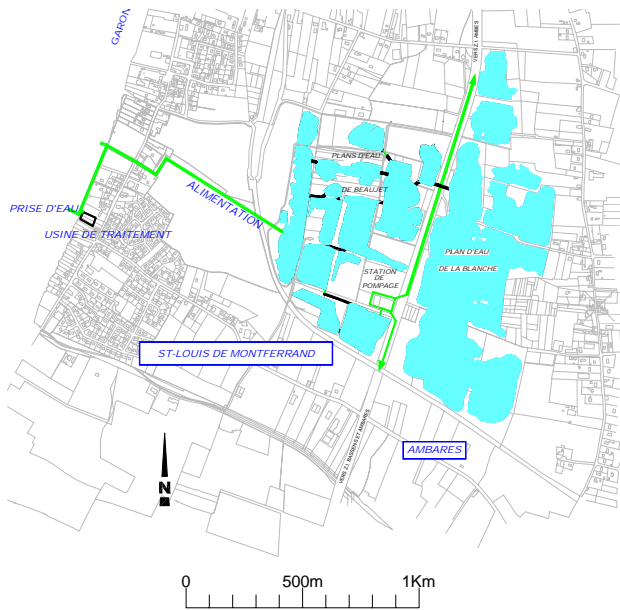
Illustration 17 : Plan des installations et vue de la prise d'eau et de l'installation de traitement de l'unité de production d'eau industrielle (CUB)
